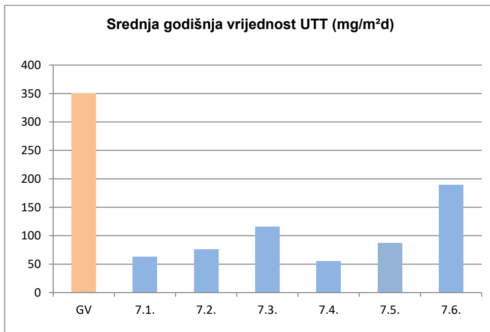
Slika 2. Raspodjela godišnjih vrijednosti UTT za 2025. god. ( \text{mg}/\text{m}^2\text{d} )
